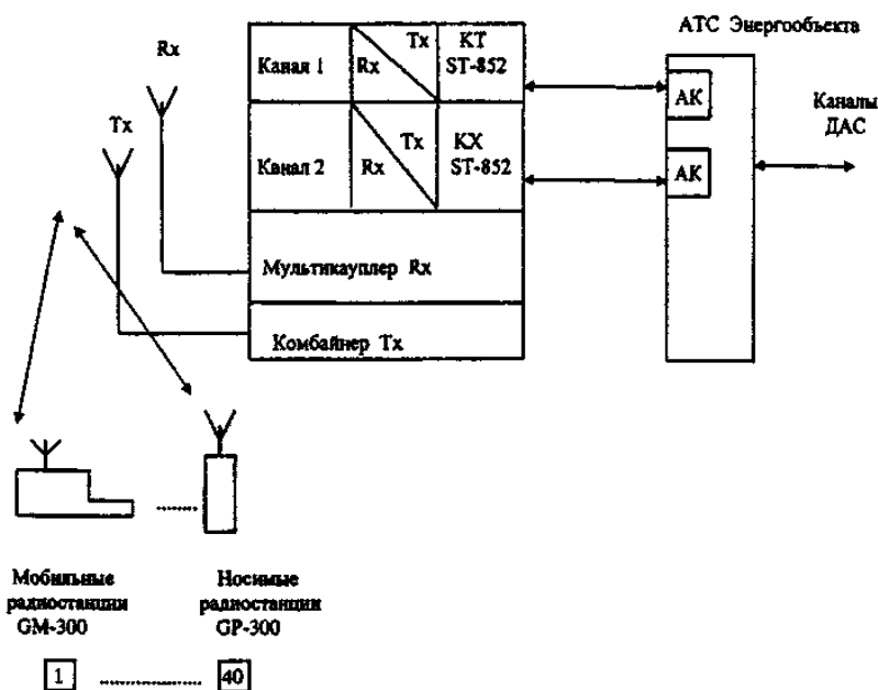
Рис. 6. Принцип организации сети транкинговой радиотелефонной связи
