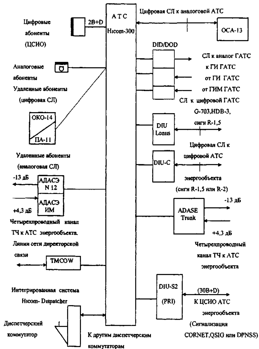
Рис. 4. Структурная схема организации ДАС с использованием АТС Nicom-300 фирмы "Siemens"
