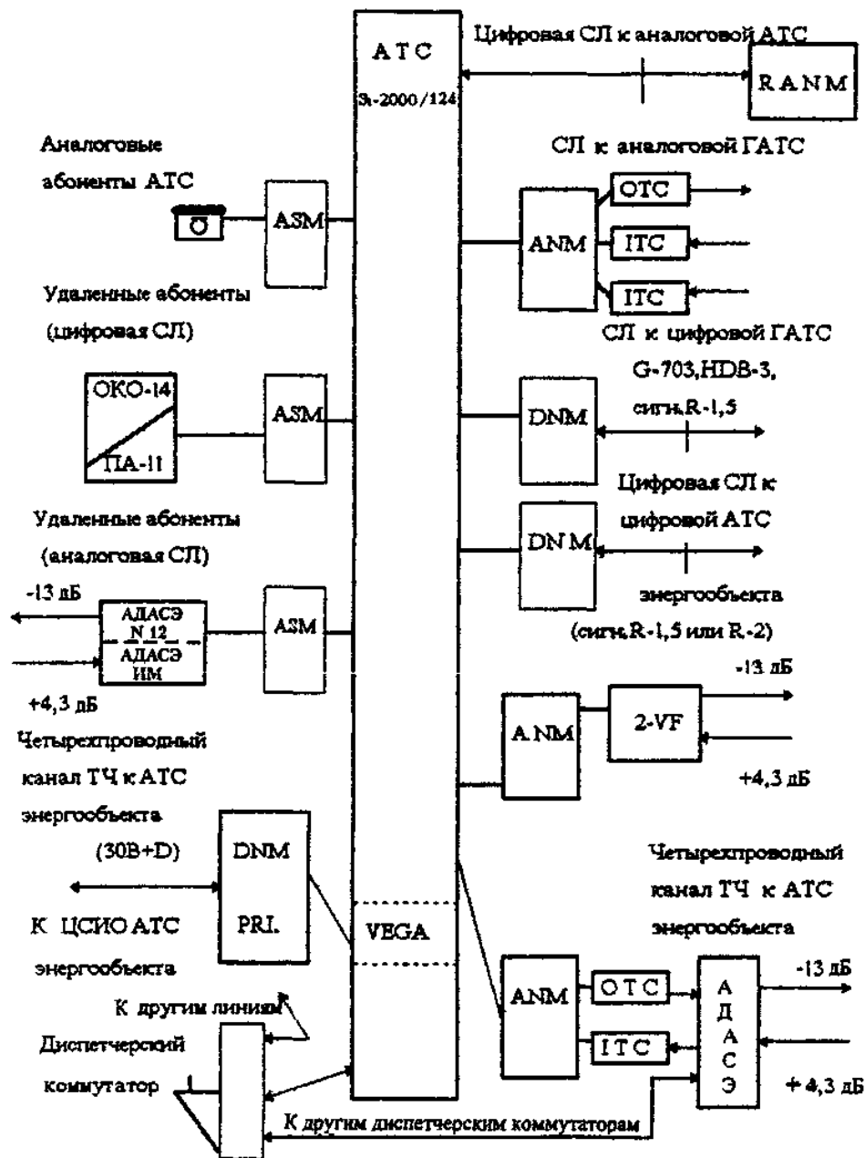
Рис. 1. Структурная схема организации ДАС с использованием цифровой АТС Si-2000/124 фирмы "Iskra"
